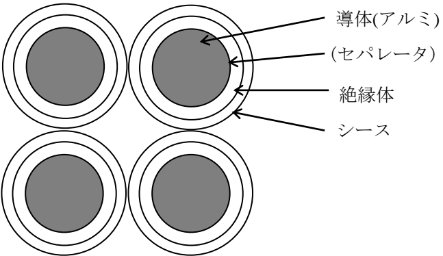
4 心 (AL-CVQ)
